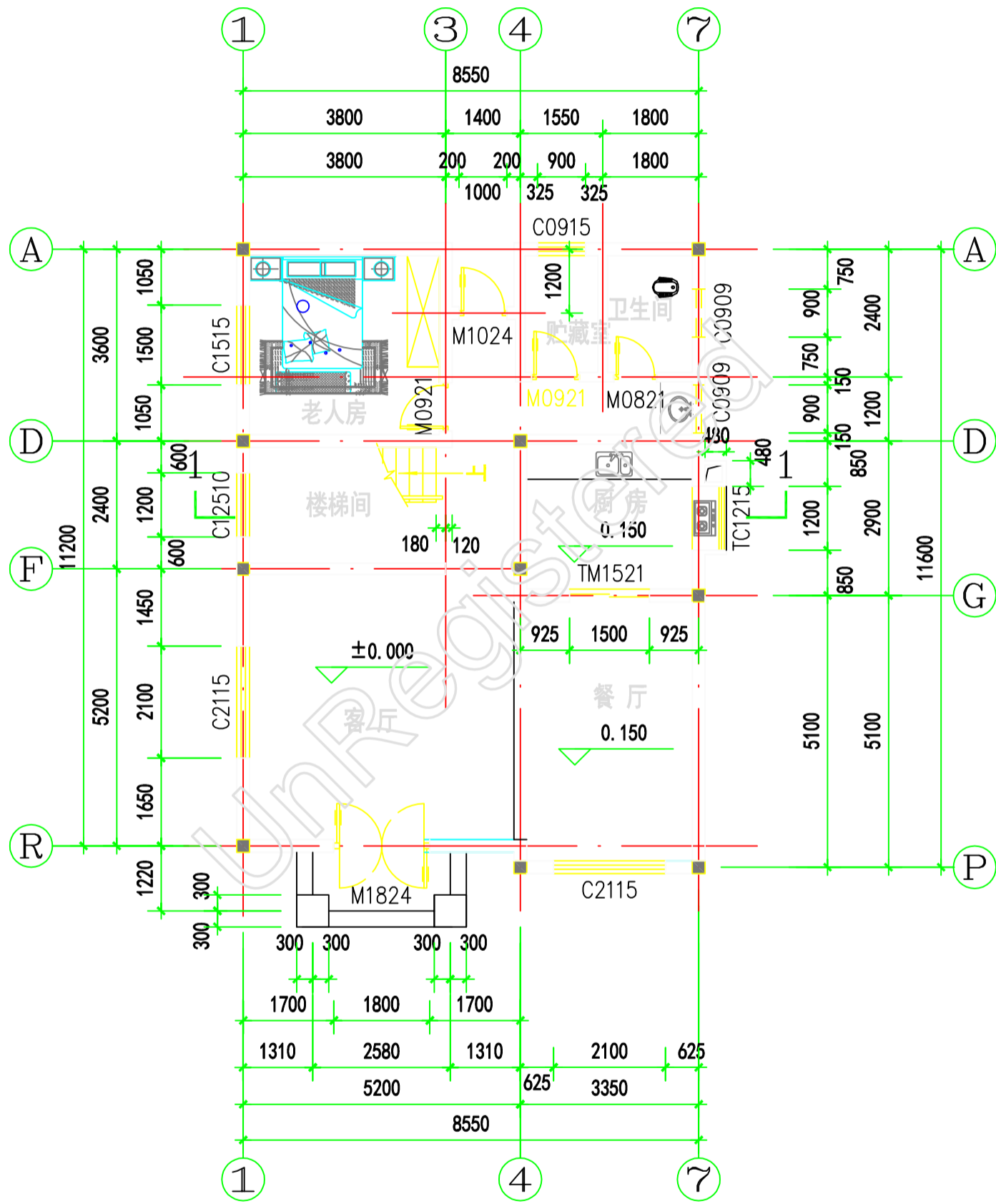
一层平面图
