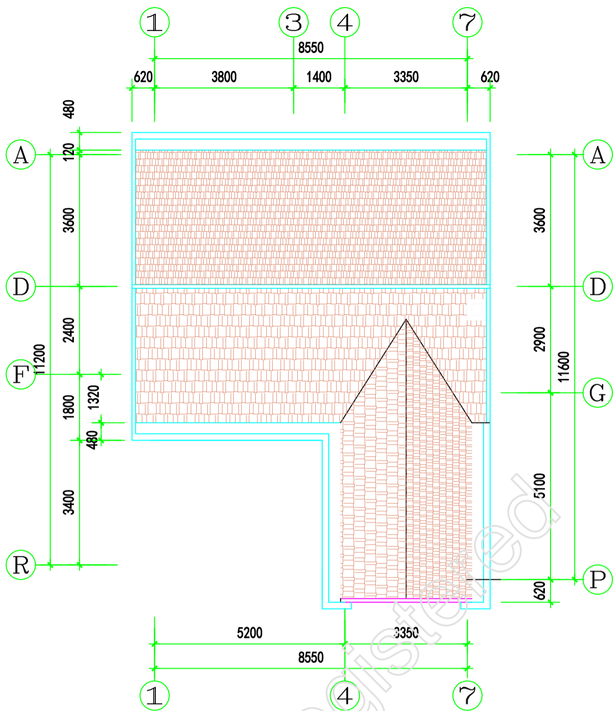
屋顶平面图
