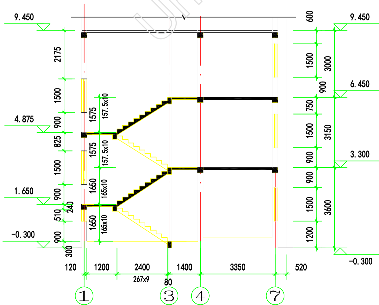
1-1剖面
