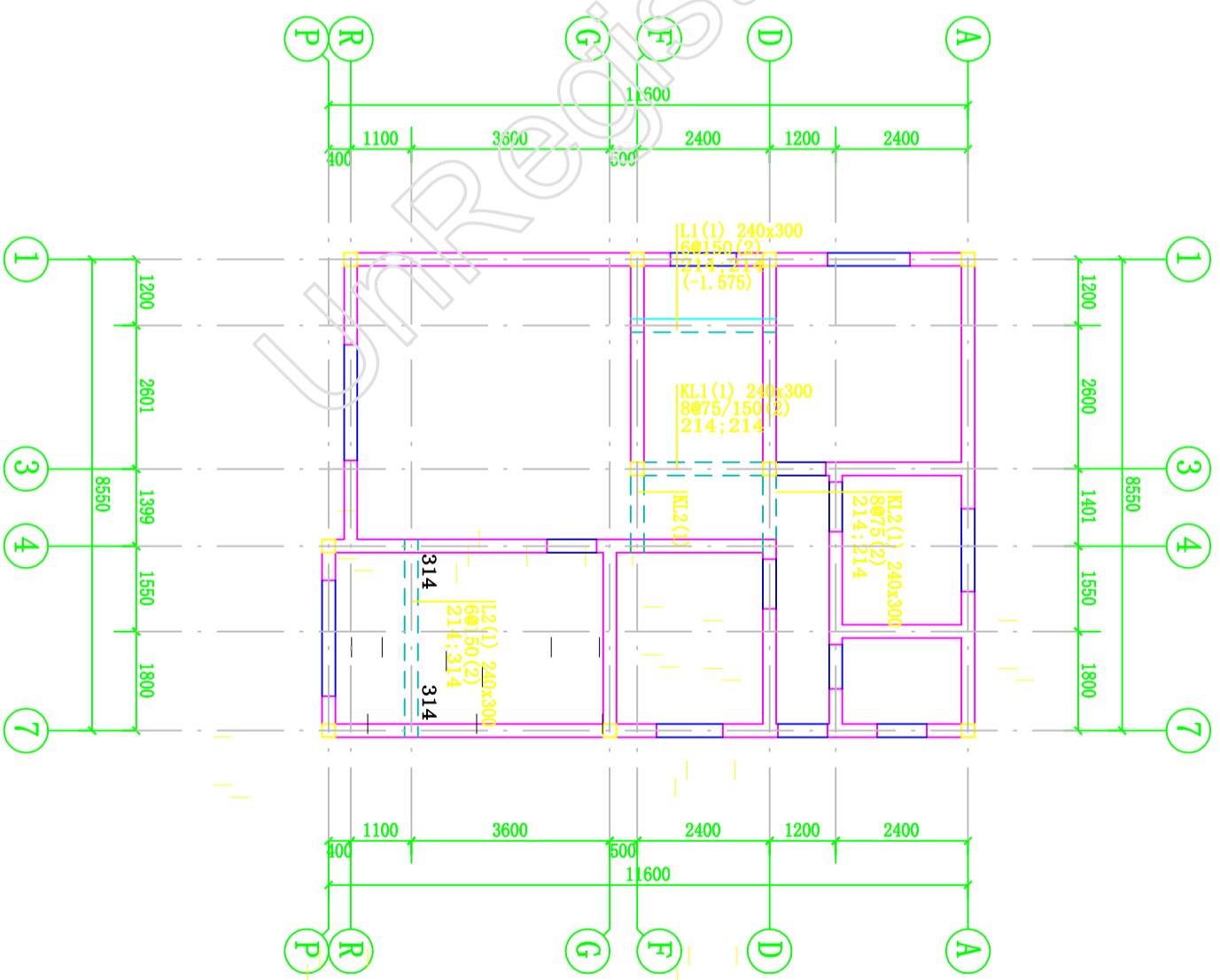
第3层梁结构平面图 1:100
