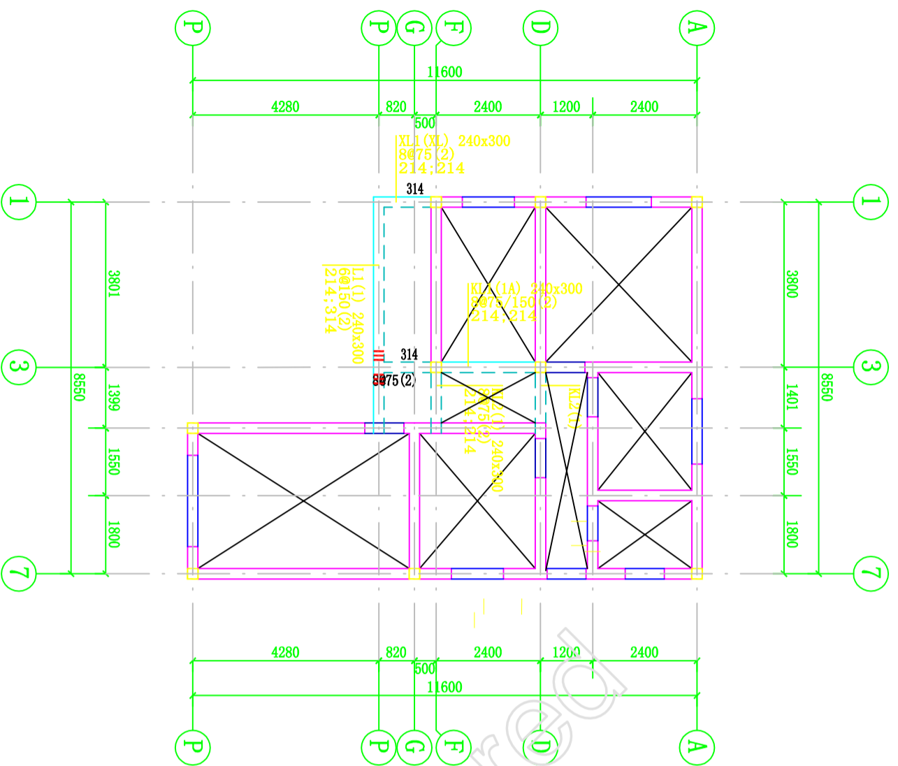
夹层梁结构平面图 1:100
