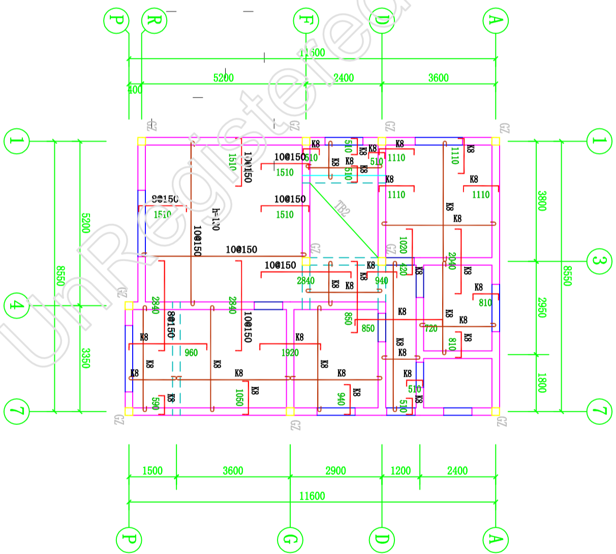
第3层结构平面图 1:100
