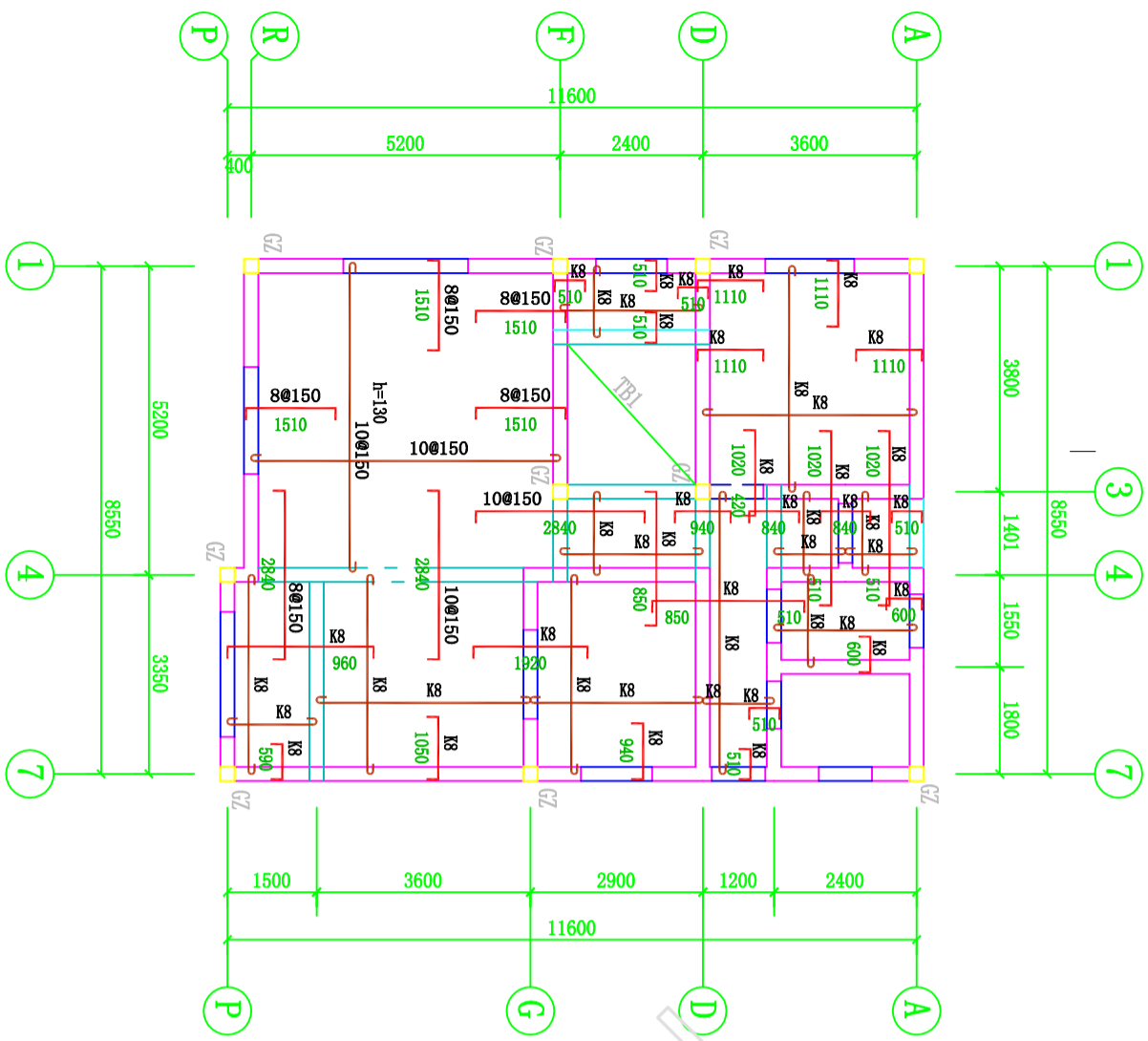
第2层结构平面图 1:100
