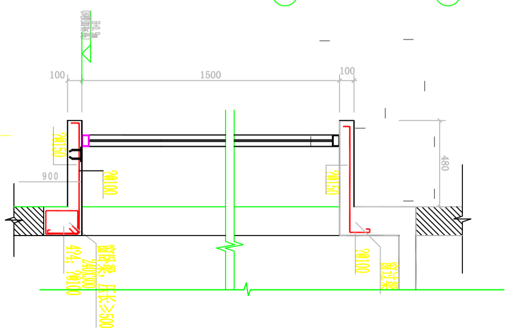
飘窗大样(C)
